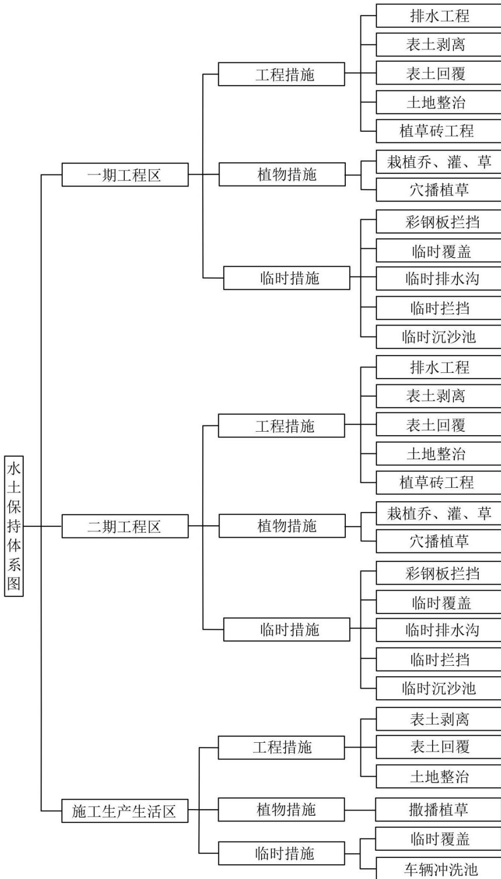
水土流失防治措施体系图
